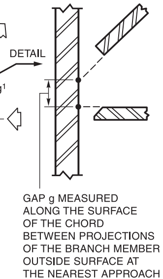
(D) Y-CONNECTION
